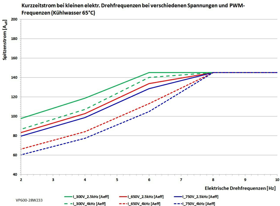
Abb: Kennlinien: Spitzenstrom für 5s über Drehfrequenz
