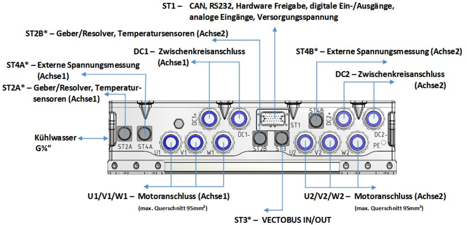
Abb: Anschlussmöglichkeiten
