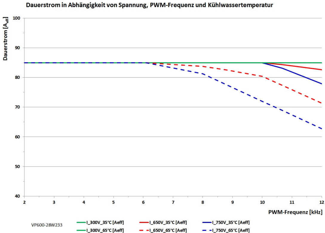
Abb: Kennlinien: Dauerstrom über PWM
