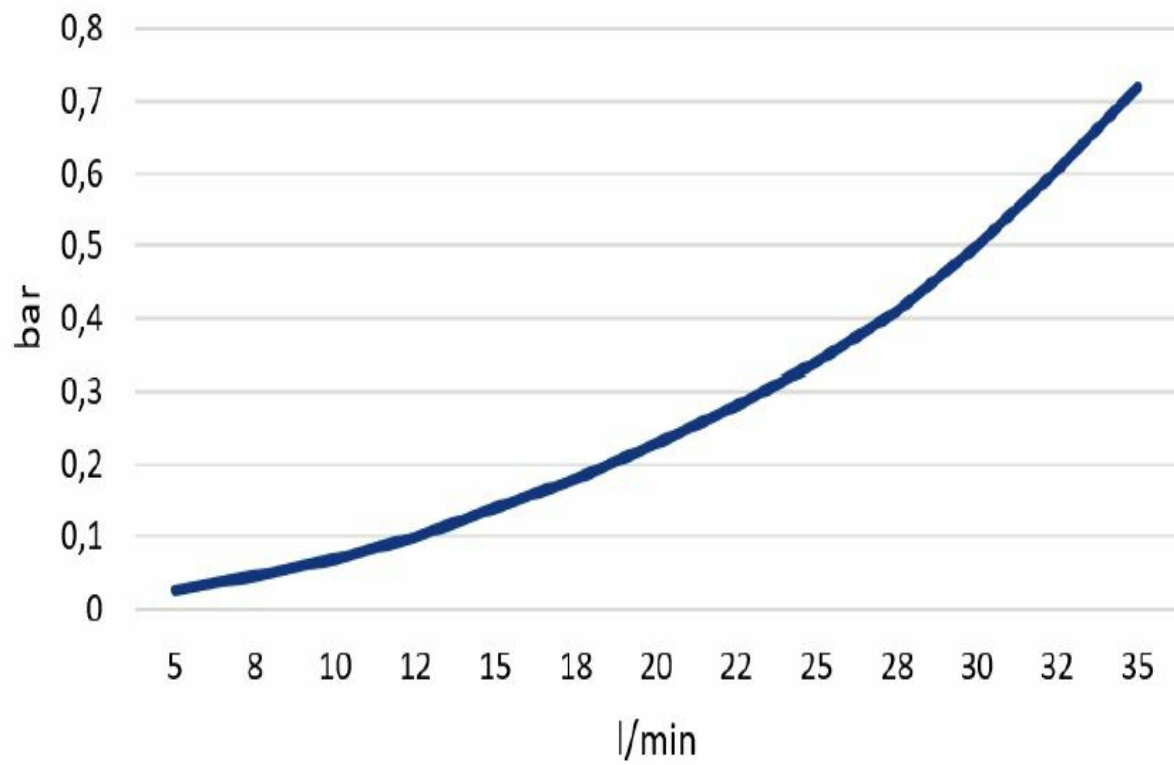
Abb: Druckverlust über Durchfluss
