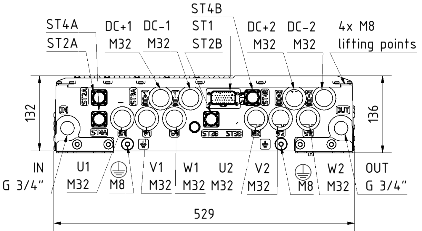
Abb: Anschlussmöglichkeiten
