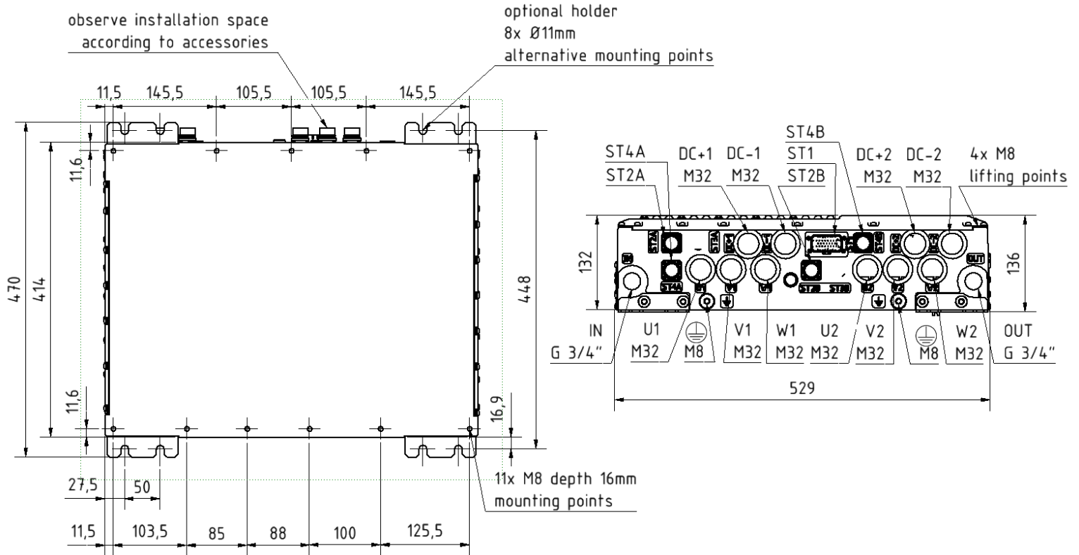
Abb: Abmessungen
