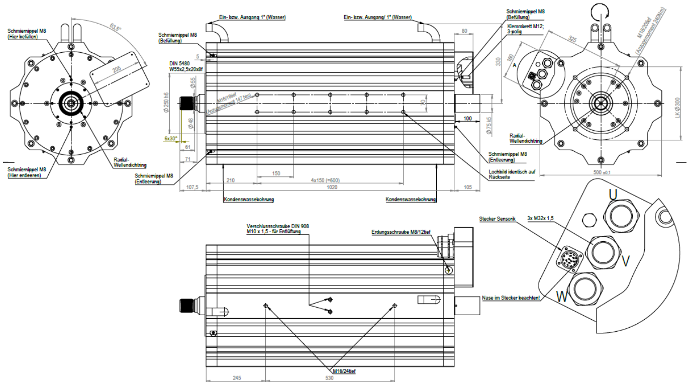
Abb: Abmessungen
